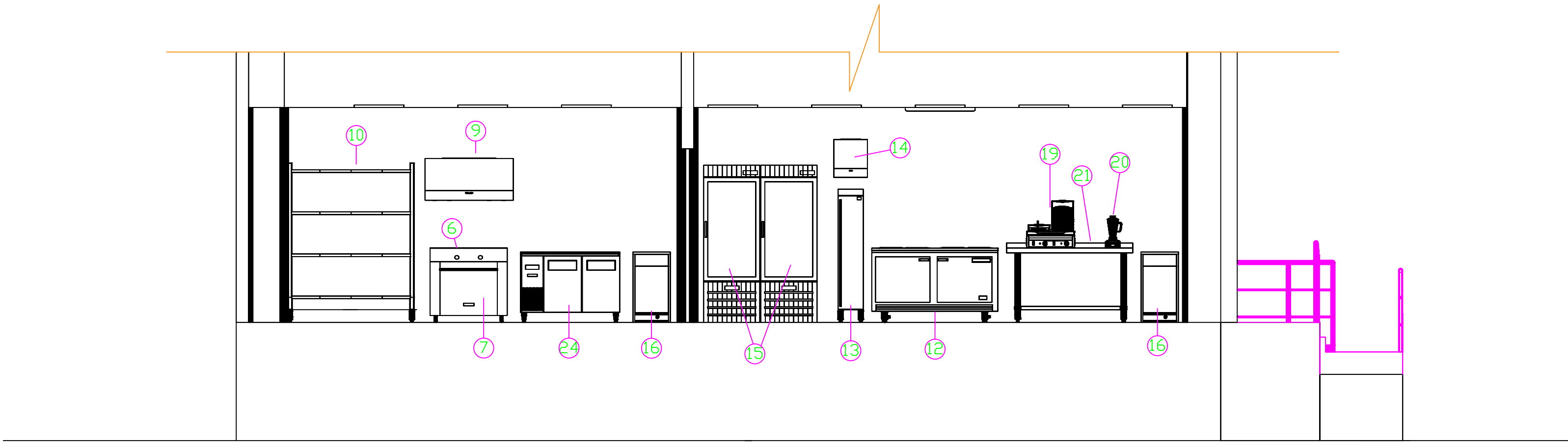
CORTE A'A''
